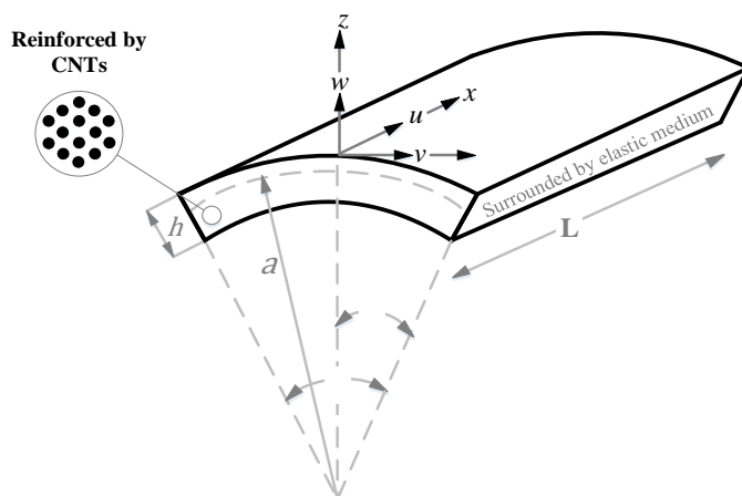
شکل ۳- شکل شماتیک المان پنل استوانه‌ای تقویت شده با نانو لوله‌ی کربنی بر بستر الاستیک با در نظر گرفتن میدان جابجایی
