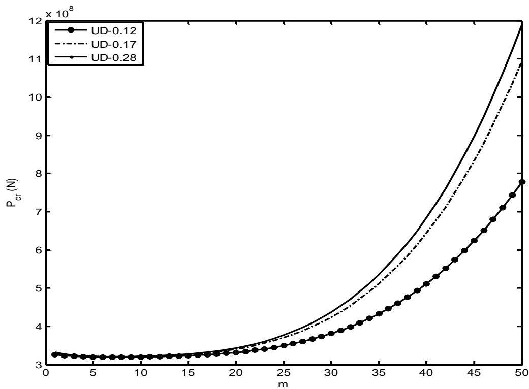
شکل ۱۰- مقایسه بار کمانش بحرانی پنل استوانه‌ای برای درصدهای مختلف نانو لوله‌های کربنی بر حسب عدد موج محیطی (n = 1, \varphi = \pi Rad, a = L = 1m, h = 0.01m, K_G = 10^9 N/m, K_W = 10^9 N/m^3) .
