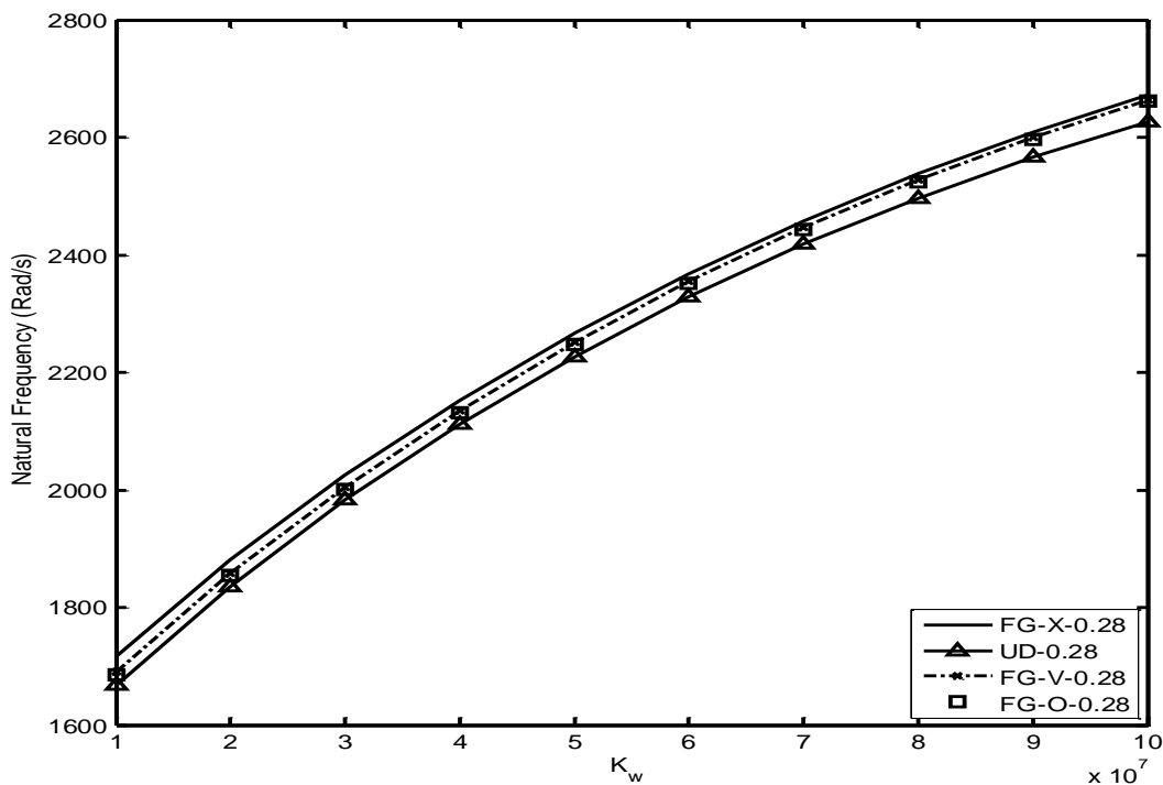
شکل ۹- نتایج مود دوم ارتعاشات پنل استوانه‌ای بر حسب K_w در توزیع‌های مختلف. (a = L = 1m, h = 0.01m, \varphi = \pi Rad)
