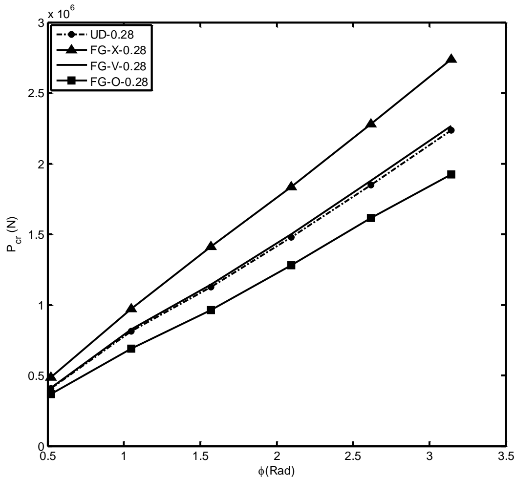
شکل ۱۲- نتایج بار کمانش بحرانی پنل استوانه‌ای بر حسب زاویه‌ی پنل ( \phi ) برای توزیع‌های مختلف نانو لوله‌های
