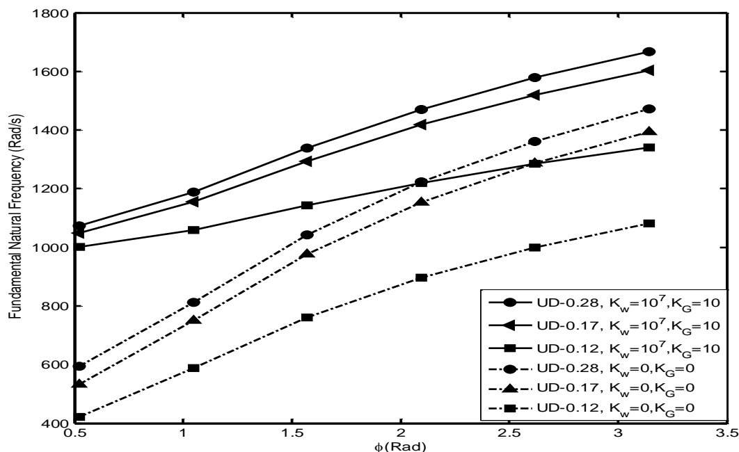
شکل ۴- نتایج مود اول (اصلی) ارتعاشات پنل استوانه‌ای بر حسب زاویه پنل ( \phi ) برای درصدهای مختلف نانولوله کربنی در
