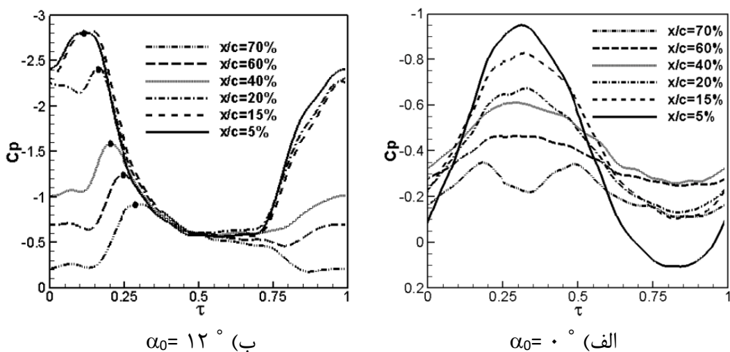
شکل ۴- تاریخچه تغییرات فشار نسبت به زمان بی بعد
