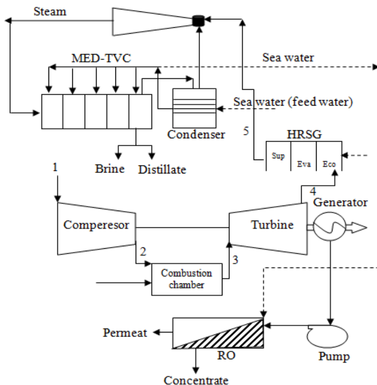
شکل ۳- شماتیک سامانه تولید همزمان
