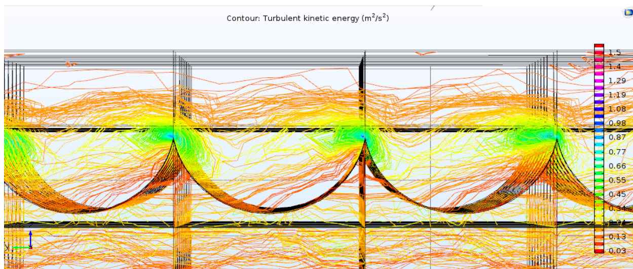
شکل ۱۱- توزیع انرژی جنبشی آشفته در صفحه y-z در مبدل حرارتی خمیده
