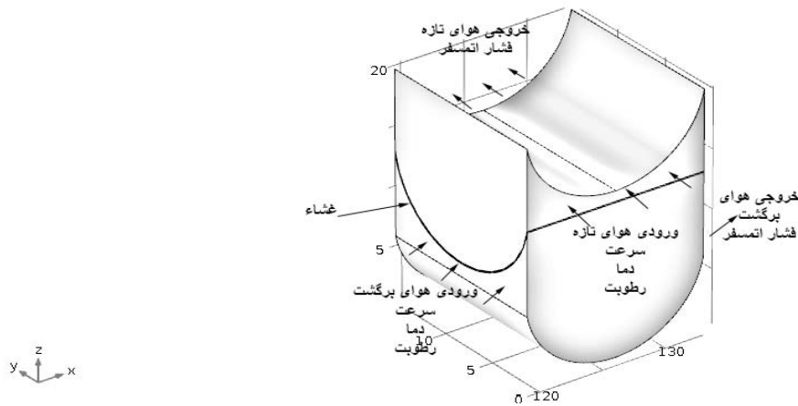
شکل ۲- شماتیک شرایط مرزی ورودی و خروجی بر روی مبدل حرارتی خمیده
