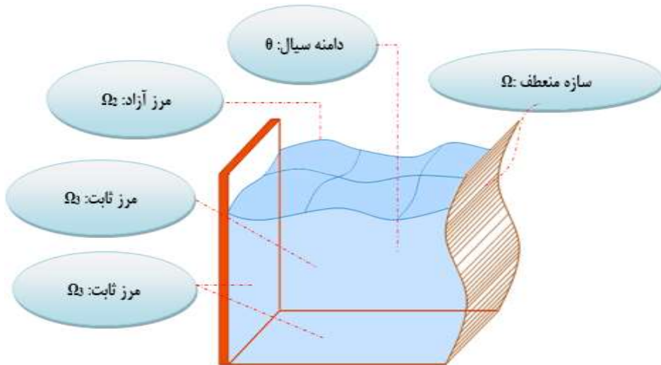
شکل ۱- شماتیک مسئله سیال - سازه و شرایط مرزی
