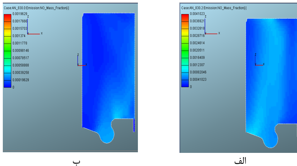
شکل ۱۰- مقایسه اکسید نیتروژن خروجی در طول پاشش ۱۲ درجه و ۵ درجه (الف) اکسید نیتروژن خروجی در طول پاشش ۵ درجه (ب) اکسید نیتروژن خروجی در طول پاشش ۱۲ درجه
