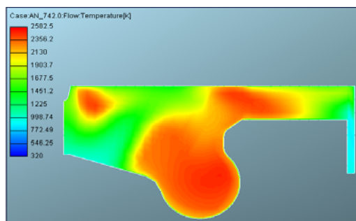
شکل ۷- حداکثر دما در طول پاشش ۱۲ درجه (حداکثر دما در طول پاشش ۱۲ درجه ۲۰۰۶ کلوین است)
