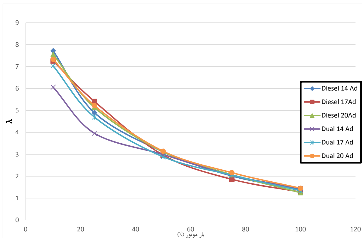
شکل ۶ - مربوط میزان لاندا در بارها و زوایای آوانس مختلف پاشش سوخت آتش زن
