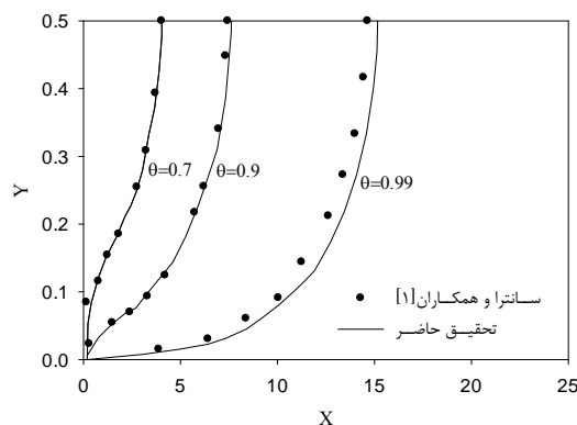
شکل ۳- اعتبارسنجی برنامه حاضر با نتایج مرجع [۱] (خطوط همدمای در \phi=0.03 و Re=10 ).
