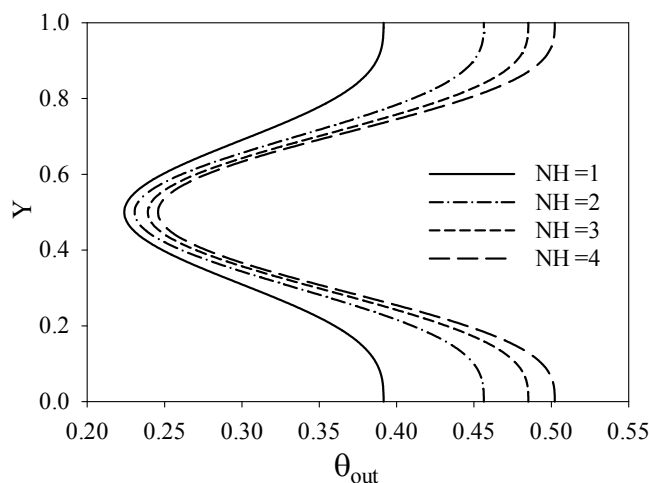
شکل ۱۴ - نمودار دمای بی‌بعد در مقطع خروجی کانال برای تعداد مختلف Re=100 ، \phi=0.03
