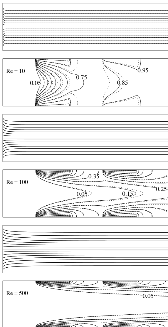
شکل ۴ - خطوط جریان (بالا) و خطوط همدم (پایین) برای نانوسیال آب - مس با \phi=0.03 (—) و آب خالص (.....) در اعداد رینولدز مختلف
