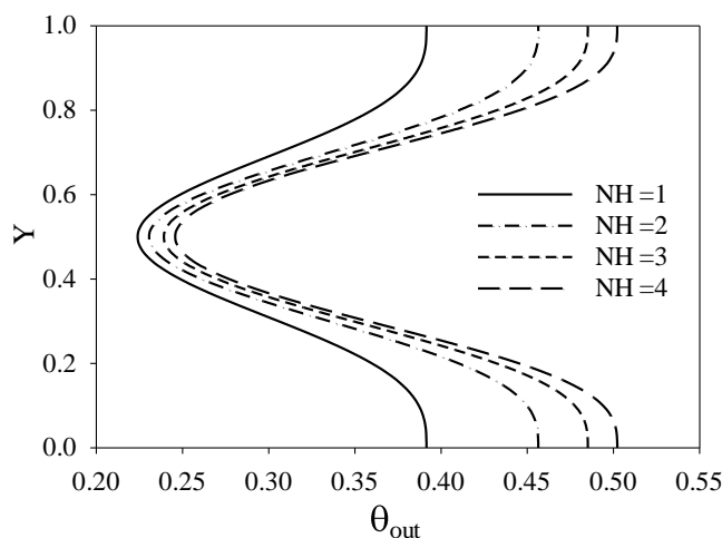
شکل ۱۴ - نمودار دمای بی‌بعد در مقطع خروجی کانال برای تعداد مختلف حرارتی در Re=100 ، \phi=0.03
