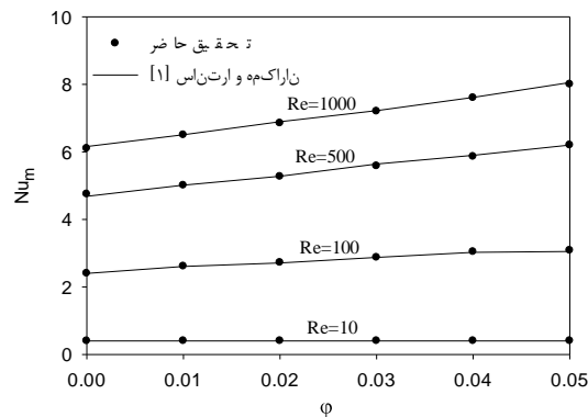
شکل ۲ - اعتبارسنجی برنامه حاضر با نتایج مرجع [۱]
