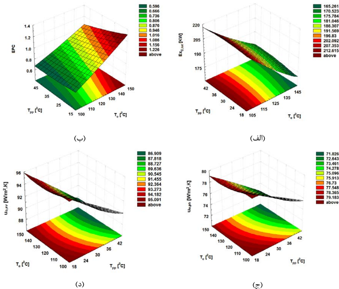
شکل ۴- تاثیر T_{pp} و T_e بر (الف) تخریب اگزرژی کل ORC، (ب) ضریب عملکرد اگزرژی ORC، (ج) ضریب انتقال حرارت کلی پیش گرمکن و (د) ضریب انتقال حرارت کلی تبخیرکن
