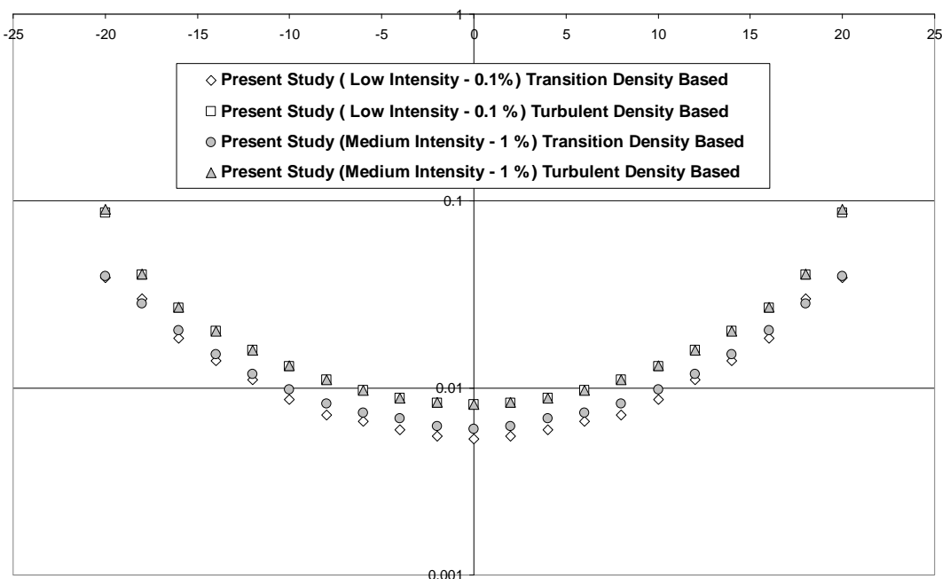
شکل ۲۴ - نمودار اختلاف میان نتایج ضریب پسا (محور عمودی) بر حسب زاویه حمله (محور افقی) - به دست آمده از تحلیل میدان جریان با استفاده از مدل قدرتمند تماماً آشفتۀ K\omega -SST نسبت به نتایج ضریب برای تحلیل میدان جریان با استفاده از مدل گذار K\omega -Transition در دو تحلیل جریان دارای سطح اغتشاش ۱ درصدی و سطح اغتشاش ۰/۱ درصدی
