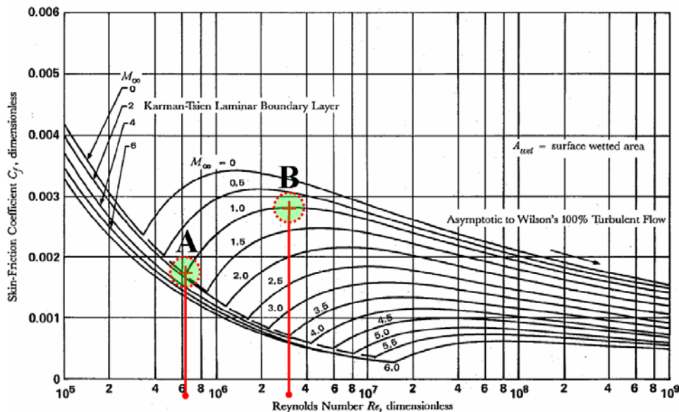
شکل ۴ - شمایکی از وابستگی طول ناحیه گذار (فاصله میان نقاط A تا B) به عدد ماخ جریان آزاد برای جریان عبوری از روی یک صفحه تخت؛ به افزایش این طول در اعداد ماخ بالاتر توجه نمایید [۱].
