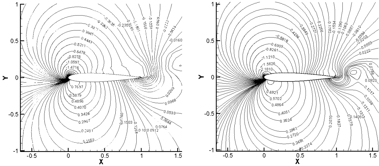
شکل ۱۹- اختلاف میان نتایج ضریب فشار C_p به دست آمده از تحلیل مدل تماماً آشفته K\omega -SST (شکل چپ) نسبت به نتایج تحلیل مدل نزدیک به واقعیت گذار K\omega -Transition (شکل راست)؛ در هر دو تحلیل در زاویه حمله 20^\circ درجه و عدد رینولدز جریان آزاد 6 میلیون و تحلیل به روش بر مبنای چگالی صورت گرفته است.
