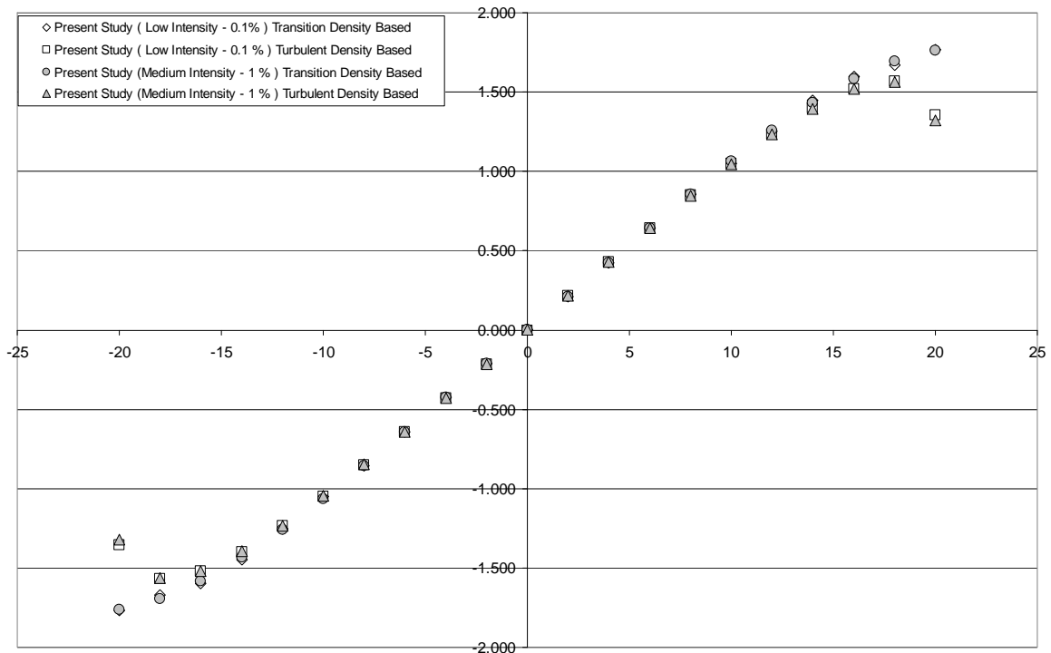
شکل ۲۲- اختلاف میان نتایج ضریب برآ بر حسب زاویه حمله - به دست آمده از تحلیل میدان جریان با استفاده از مدل قدرتمند تماماً آشفتۀ K\omega -SST نسبت به نتایج ضریب برآی تحلیل میدان جریان با استفاده از مدل گذار K\omega -Transition در دو تحلیل جریان دارای سطح اغتشاش ۱ درصدی و سطح اغتشاش ۰/۱ درصدی؛ مجدداً وقوع شرایط واماندگی پیش از موعد (یا همان واماندگی زودرس) در فرض جریان تماماً آشفتۀ مشهود است؛ در هر دو تحلیل عدد رینولدز جریان آزاد ۶ میلیون و تحلیل به روش بر مبنای چگالی صورت گرفته است.
