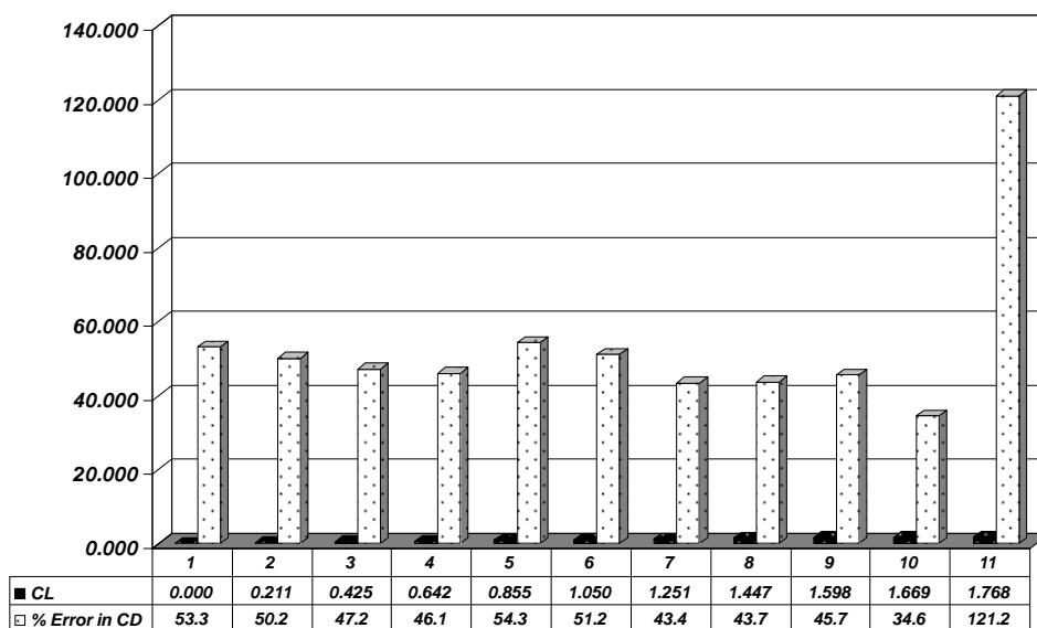
شکل ۱۵ - اختلاف میان نتایج ضریب پسای به دست آمده از مدل قدرتمند تماماً آشفتۀ K\omega -SST نسبت به نتایج مدل گذار K\omega -Transition در عدد رینولدز جریان آزاد ۶ میلیون و تحلیل به روش بر مبنای چگالی.
