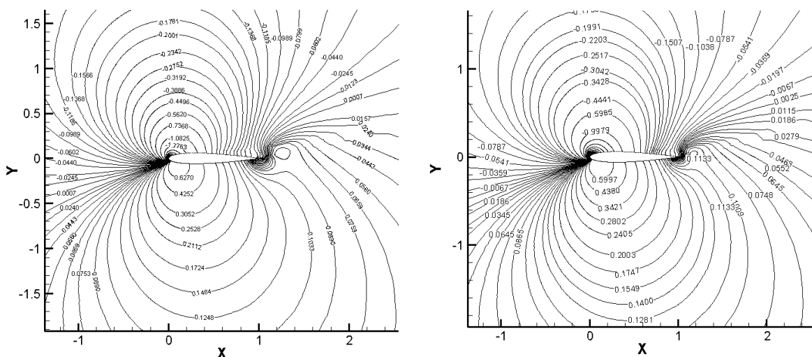
شکل ۱۷ - اختلاف میان نتایج ضریب فشار C_p به دست آمده از تحلیل مدل تماماً آشفتۀ K\omega -SST (شکل چپ) نسبت به تحلیل مدل گذار K\omega -Transition (شکل راست)؛ در هر دو تحلیل در زاویه حمله ۱۸ درجه و عدد رینولدز جریان آزاد ۶ میلیون و تحلیل به روش بر مبنای چگالی صورت گرفته است.
