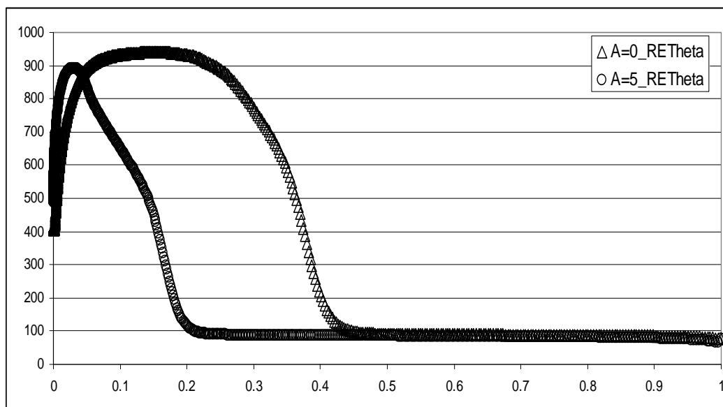
شکل ۲۷- نمودار توزیع Re_{\theta} بر روی سطح ایرفویل؛ تحت تاثیر اثرات گرادیان فشار معکوس، وقوع گذار در زاویه حمله ۵ درجه نسبت به زاویه حمله صفر درجه تسریع یافته است.
