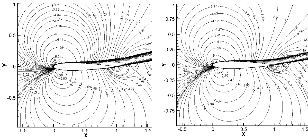
شکل ۱۸ - اختلاف میان نتایج توزیع سرعت به دست آمده از تحلیل مدل تماماً آشفتۀ K\omega -SST (شکل چپ) نسبت به مدل گذار K\omega -Transition (شکل راست)؛ در هر دو تحلیل در زاویه حمله ۱۸ درجه و عدد رینولدز جریان آزاد ۶ میلیون و تحلیل به روش بر مبنای چگالی صورت گرفته است.
