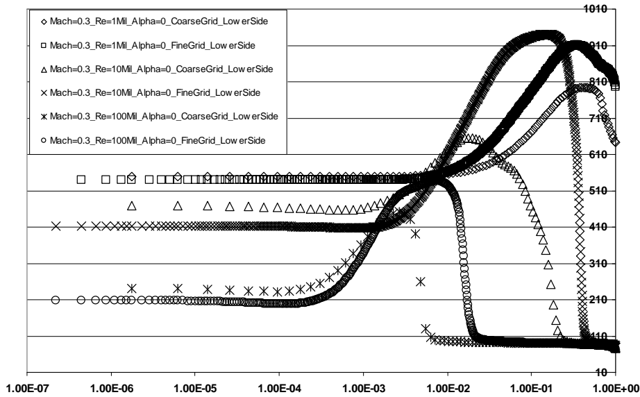
شکل ۳۵- تغییرات عدد رینولدز ضخامت منبسط Re_0 در عدد ماخ 0.3 و زاویه حمله صفر در اعداد رینولدز طولی مختلف و تراکمهای شبکه های محاسباتی مختلف (به منظور نمایش بهتر نتایج، نمودار افقی نیمه لگاریتمی ترسیم شده است)
