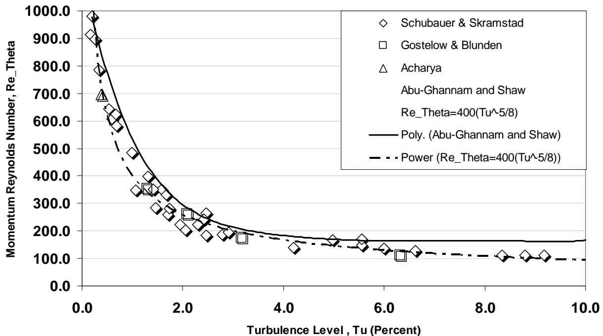
شکل ۶ - شماتیکی مقایسه میان رابطه ارائه شده توسط مایل و رابطه ارائه شده توسط ابوغنم و شاو و پراکندگی مقادیر اندازه گیری شده توسط دیگر محققین در اطراف این دو رابطه [۹]
