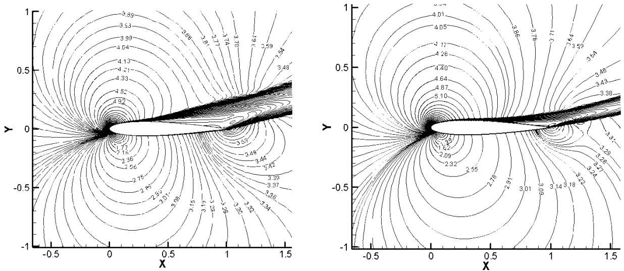
شکل ۲۰- اختلاف میان نتایج توزیع سرعت به دست آمده از تحلیل مدل تماماً آشفته K\omega -SST (شکل چپ) نسبت به نتایج تحلیل مدل نزدیک به واقعیت گذار K\omega -Transition (شکل راست)؛ در هر دو تحلیل در زاویه حمله 20^\circ درجه و عدد رینولدز جریان آزاد 6 میلیون و تحلیل به روش بر مبنای چگالی صورت گرفته است.
