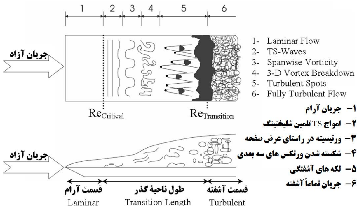
شکل ۱- شماتیکی از فرآیند گذار طبیعی که توسط شلیختینگ و در سال (۱۹۷۹) به تصویر کشیده شده است؛ به عنوان استفاده شده برای هر مرحله و نیز معیارهای Re_{Critical} (نقطه ظهور امواج تولمین - شلیختینگ ۱ T-S) و Re_{Transition} (نقطه اتمام فرآیند گذار) قید شده بر روی شکل توجه نمایند. همانطور که مشاهده می شود، امواج T-S تنها به مراحل میان ظهور تا رشد اولیه امواج تشکیل شده در جریان اطلاق شده و به هیچ عنوان شامل مراحل بعدی رشد امواج اغتشاشی نخواهند بود [۸].
