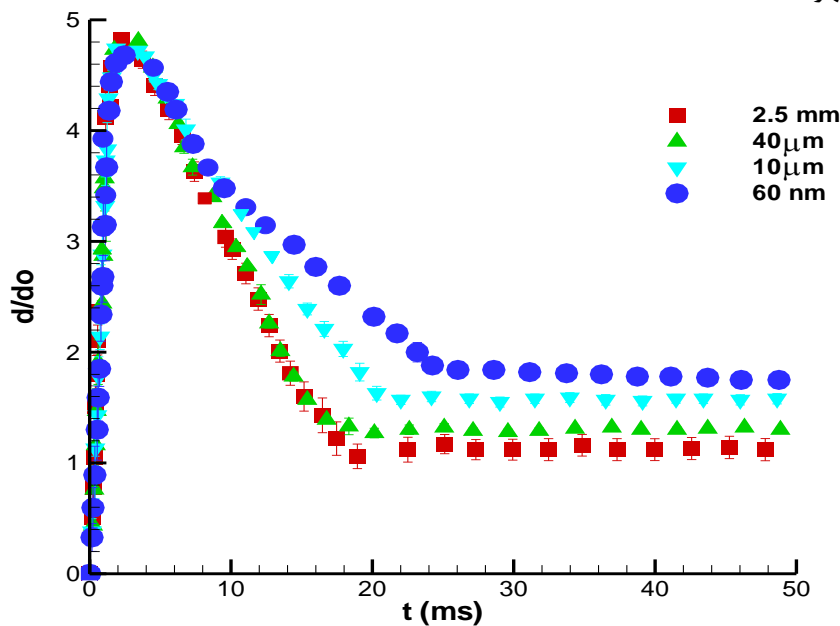
شکل ۵- ارزیابی قطر ترشوندگی آب بر روی سطح PDMS 1:40 در ضخامت های مختلف فیلم و سرعت برخورد V_0 = 5 \text{ m/s}
