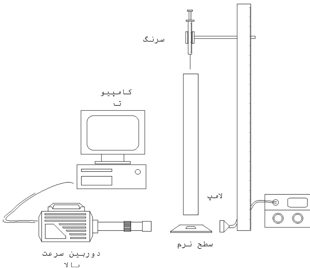
شکل ۱- دستگاه آزمایش
