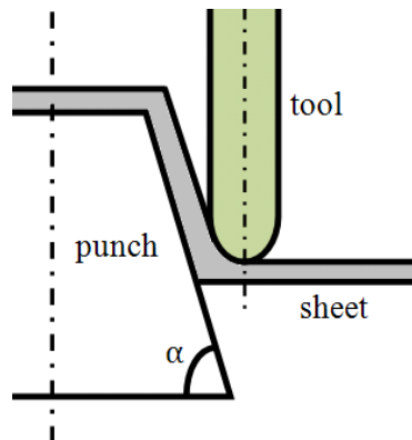
شکل ۲- ورق مخروطی
