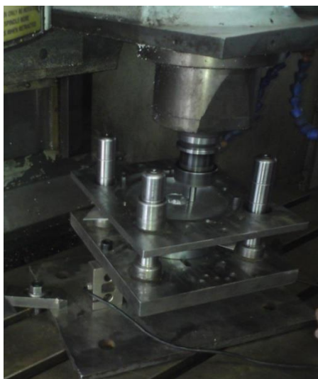
شکل ۸- تجهیزات آزمایشگاهی (CNC، قالب، ورق، ابزار، لودسل و ...)
