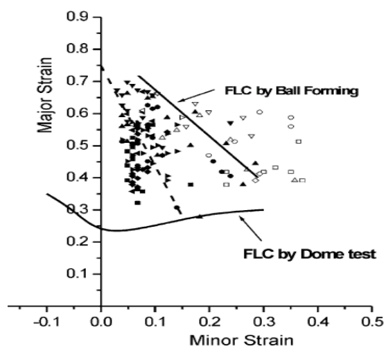
شکل ۱- نمودار محدوده فرم دهی [۷]
