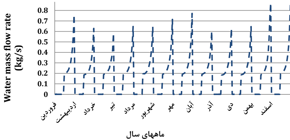
شکل ۹- دبی جرمی آب تزریقی به مبدل در طول سال، بطور متوسط ماهیانه ساعتی
