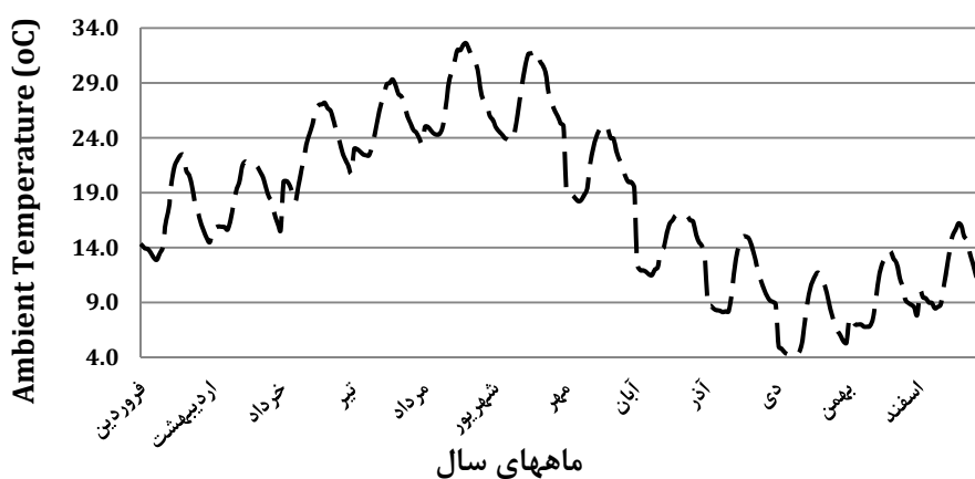
شکل ۴- دمای محیط شهر آزادشهر در سال ۱۳۹۰ بصورت متوسط ماهیانه ساعتی
