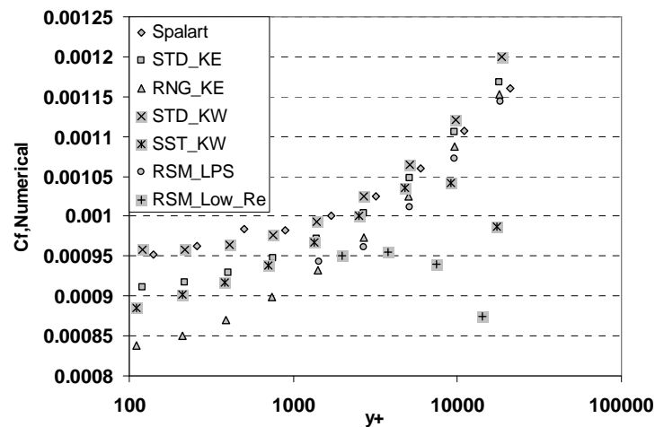
شکل ۵- نتایج حاصل از تحلیل لایه مرزی مافوق صوت در عدد رینولدز ۸۲۷ میلیون و عدد ماخ ۲/۸۳۱
