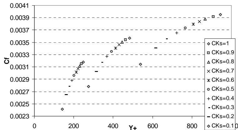
شکل ۱۸- تغییرات C_f بر حسب y^+ ( به دست آمده از مدل آشفتهگی K- \omega SST ) برای لایه مرزی با عدد ماخ جریان آزاد برابر 2/73 و عدد رینولدز 20 میلیون و دمای دیواره 273 کلین و K_s^+=104
