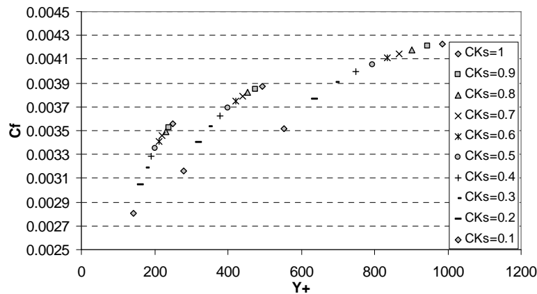
شکل ۱۹- تغییرات C_f بر حسب y^+ ( به دست آمده از مدل آشفتهگی K- \omega SST ) برای لایه مرزی با عدد ماخ جریان آزاد برابر 2/7 و عدد رینولدز 20 میلیون و دمای دیواره 273 کلین و K_s^+=571
