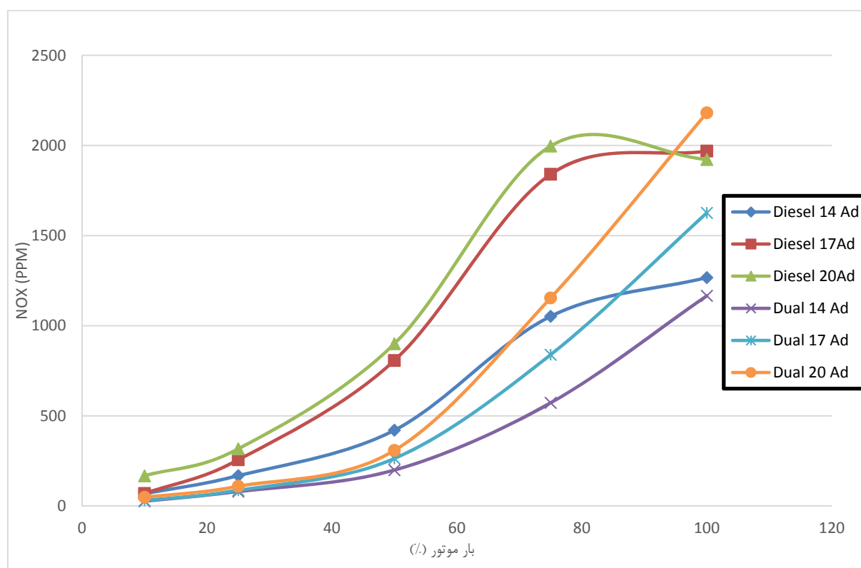
شکل ۴ - نمودار مربوط آلاینده NOx در بارها و زوایای آوانس پاشش سوخت آتش زن
